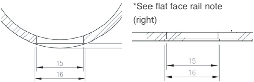
Curved Face (Tube) Rail
