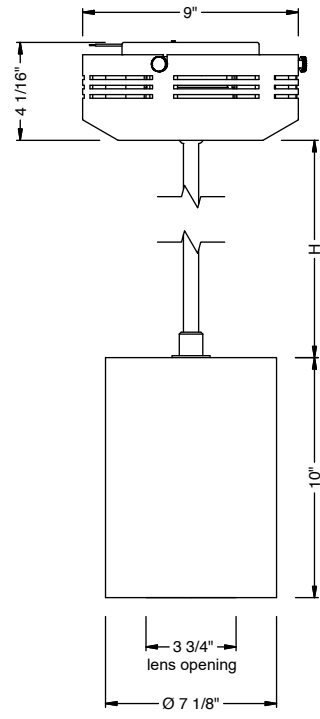
RP Rigid Pendant
