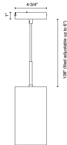
PENDANT ELV1 / CAS CANOPY
