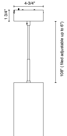
PENDANT DIM10 CANOPY
